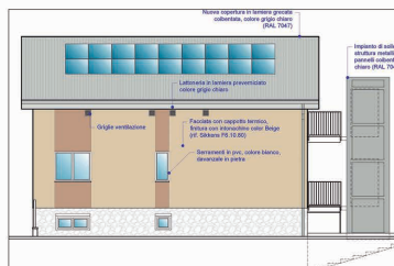
Prospetto OVEST Progetto - Scala 1:100
