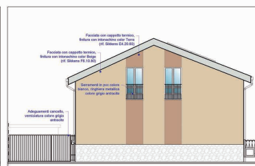
Prospetto NORD Progetto (su Via Leoncavallo) - Scala 1:100
