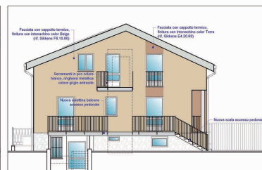
Prospetto SUD Progetto - Scala 1:100
